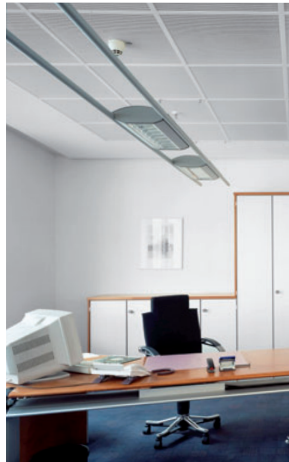
Streckmetall-Deckenverkleidung mit eingelegten Kühlmäandern
