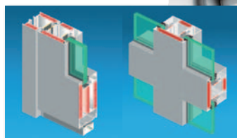
Profilschnitt Brand-schutztür und Fassade
