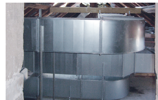
Hochwertige Lüftungstechnik auch auf engstem Raum
