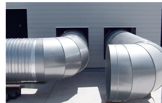
Dachauslässe geschützt gegen Korrosion und mit Vogelschutzgitter
